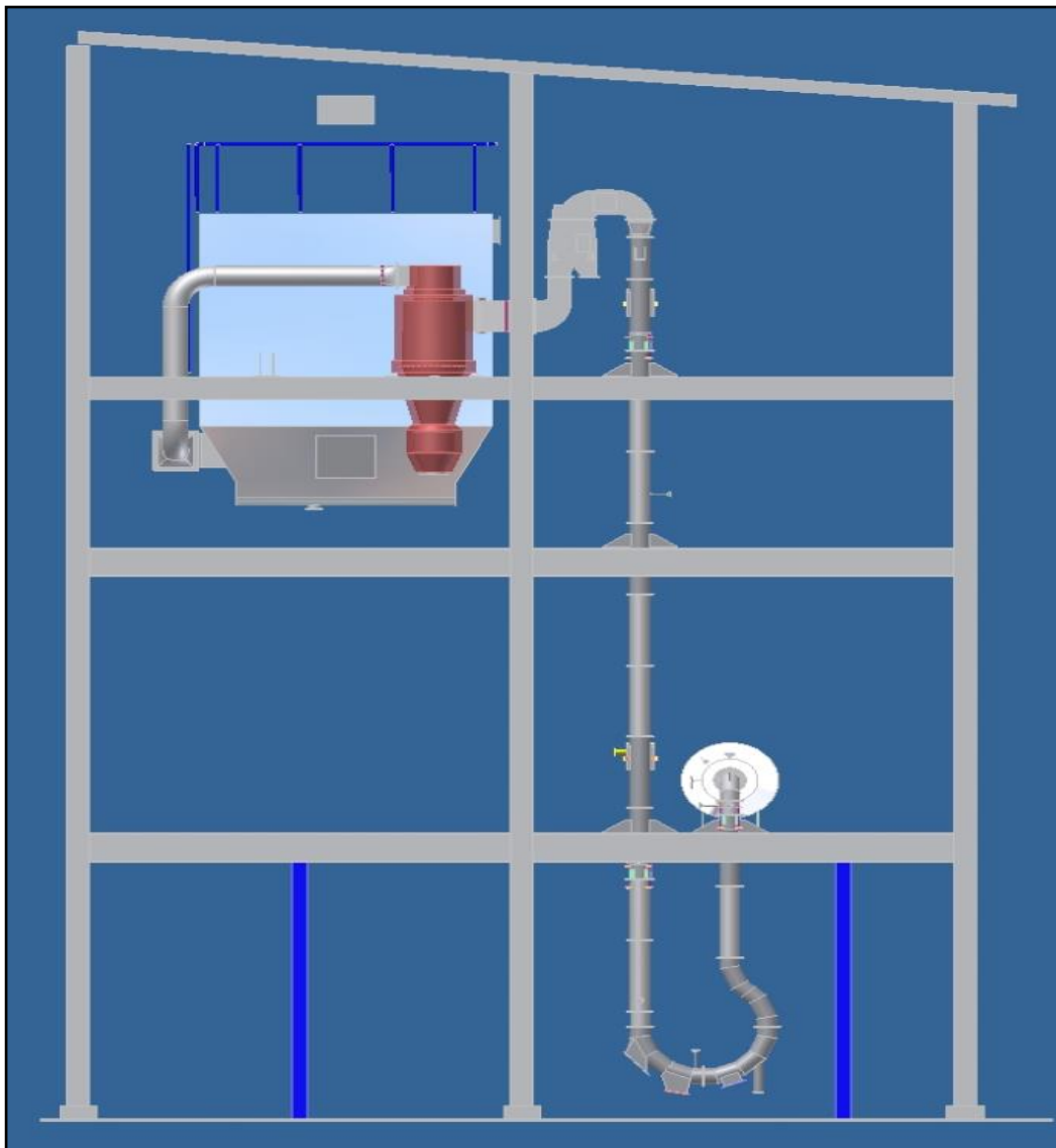
2D- Modell: Flash Dryer
